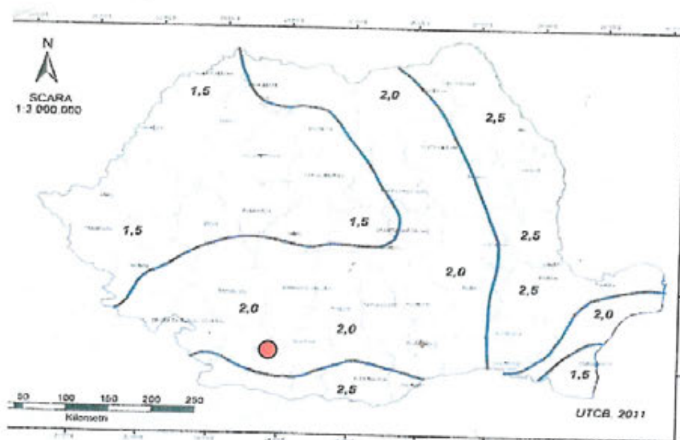
I Zonarea valorilor caracteristice ale încărcării din zapada pe sol s_k , \text{kN/m}^2 , pentru altitudini A \leq 1000 m NOTA: Pentru altitudini A > 1000 m valorile s_k se determină cu relațiile (3.1) și (3.2)
