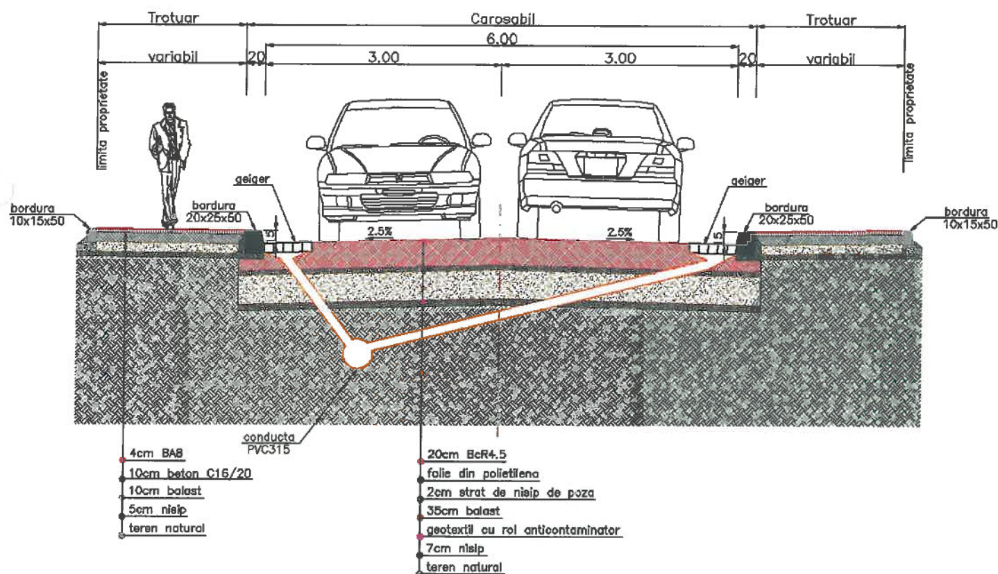
Profil transversal tip caracteristic scenariului 2
