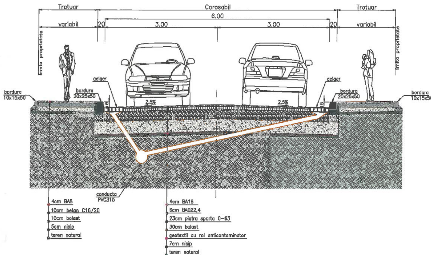
Profil transversal tip predominant
