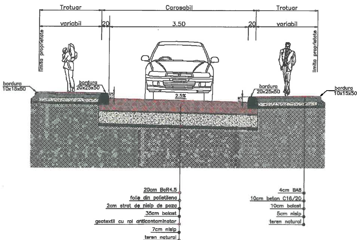
Profil transversal tip caracteristic scenariului 2
