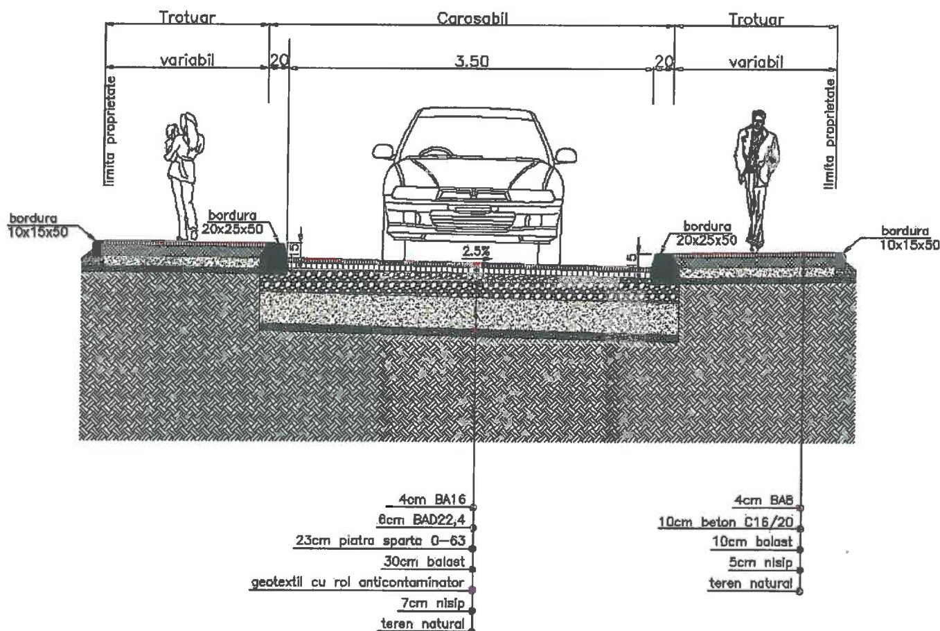
Profil transversal tip predominant
