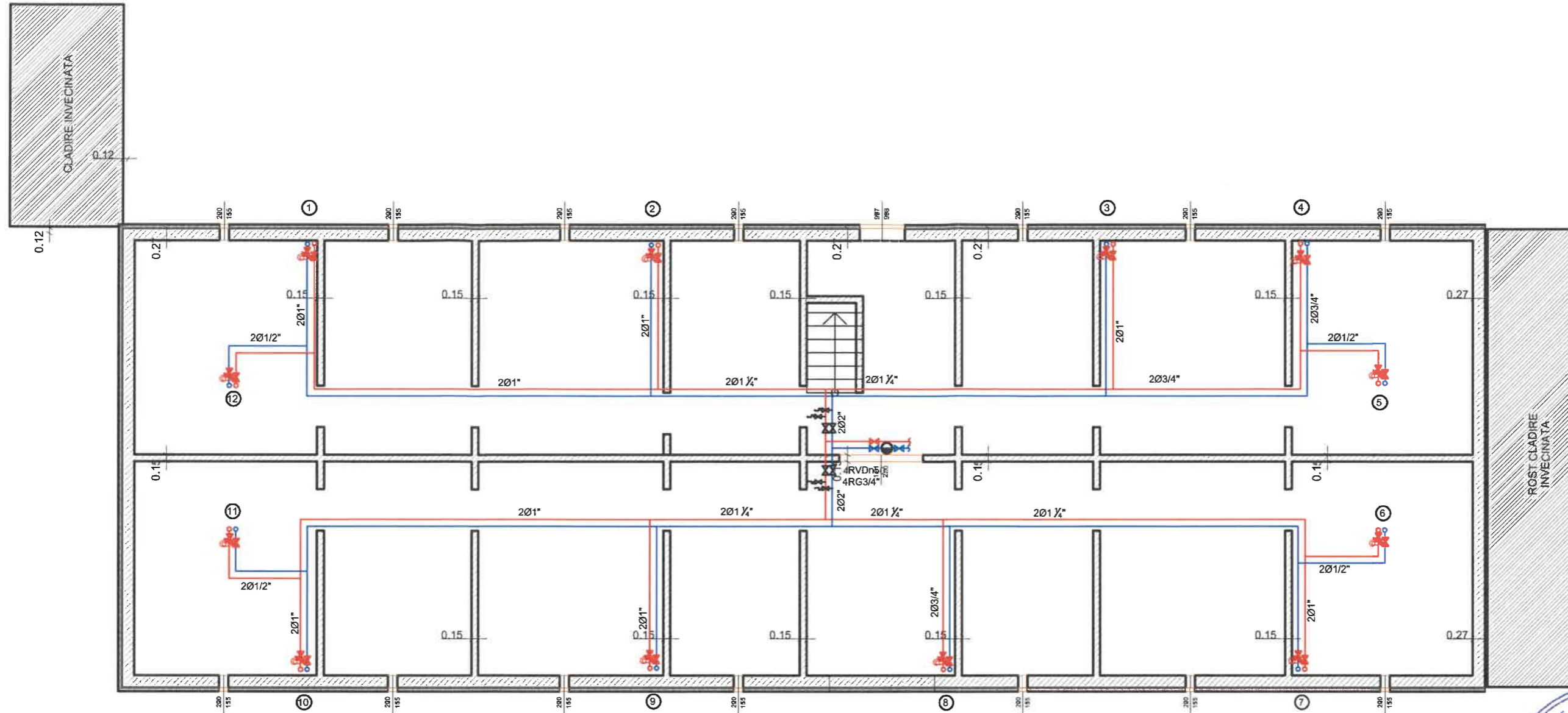
Echivalența diametrelor conductelor de încălzire OVPP-R S=2,5 SDR=6, PN20
