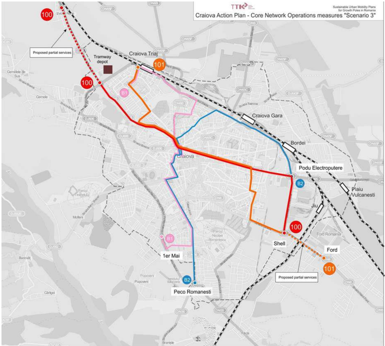
Figura 148: Măsurile propuse pentru operarea transportului public în municipiul Craiova, (linii principale)
