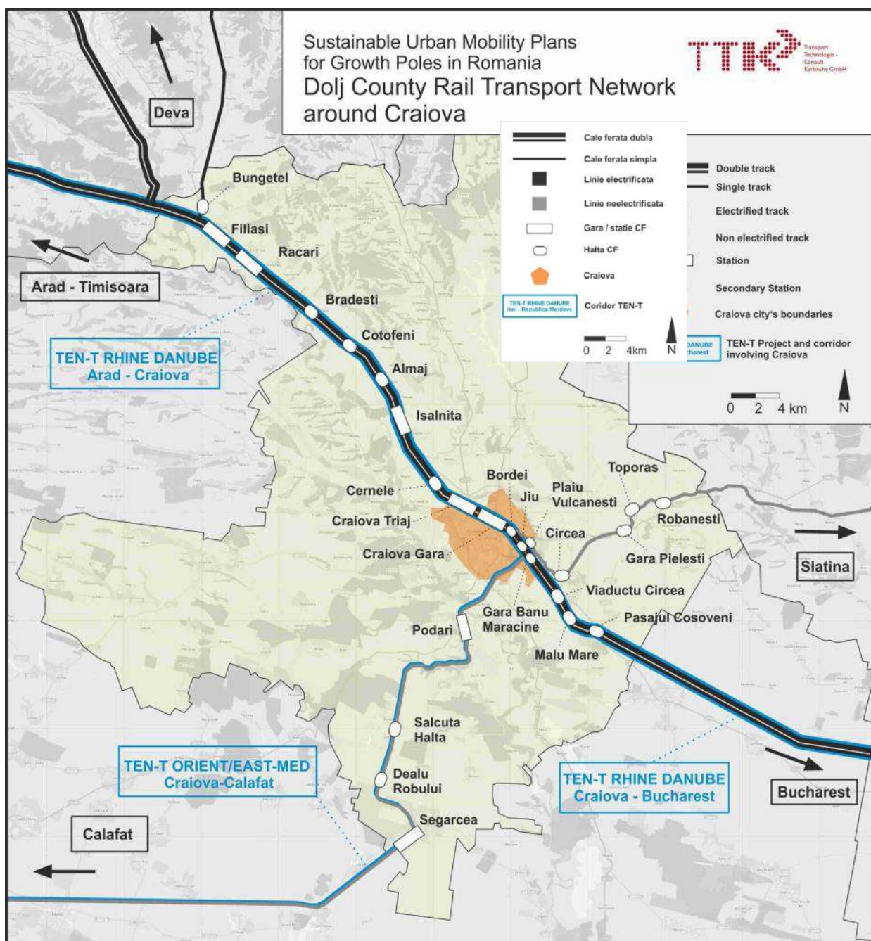
Figura 36: Rețeaua de transport pe calea ferată în jurul Craiovei
