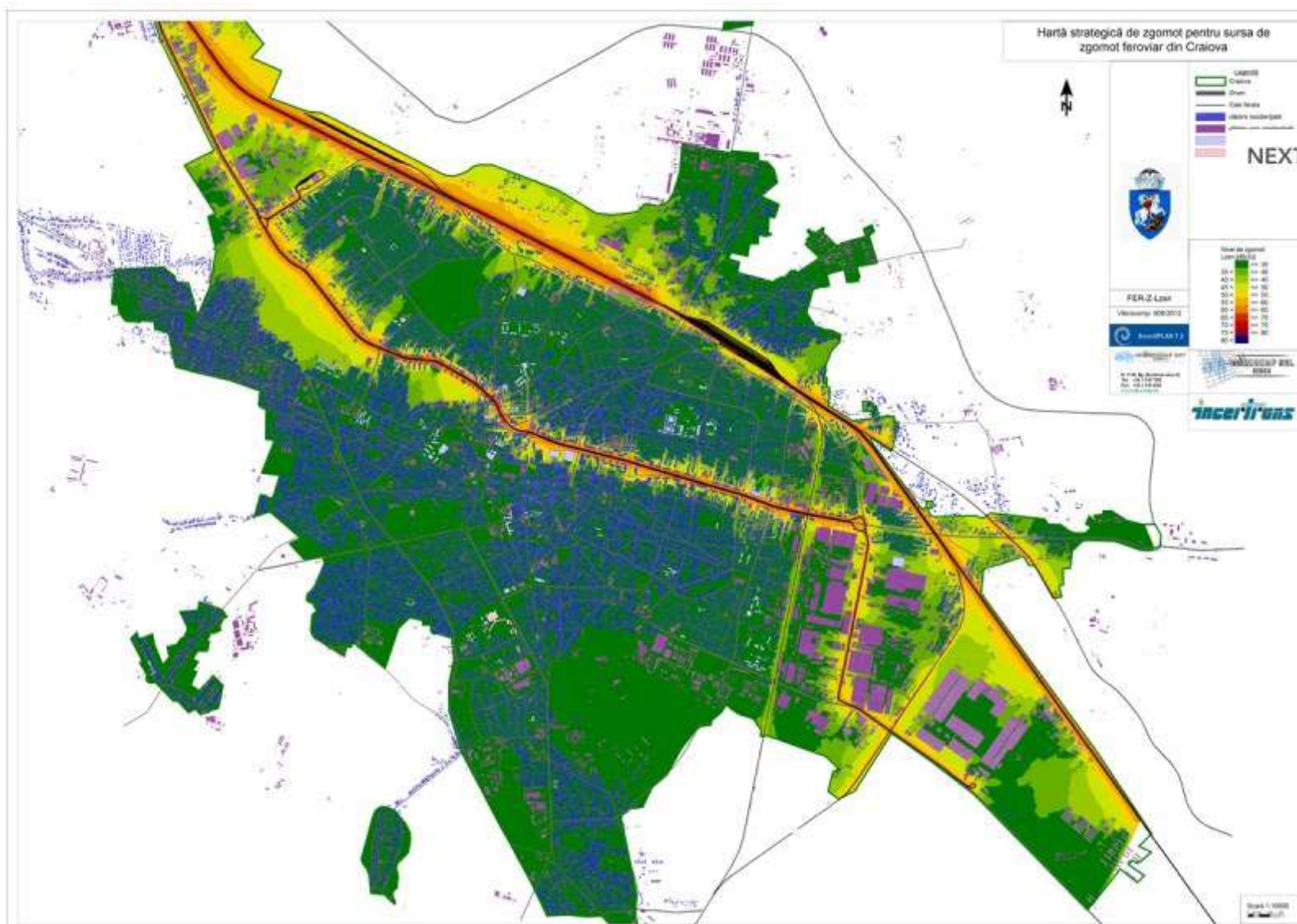
Figura 100: Aglomerarea Craiova- sursa trafic feroviar, indicatorul Lzsn
