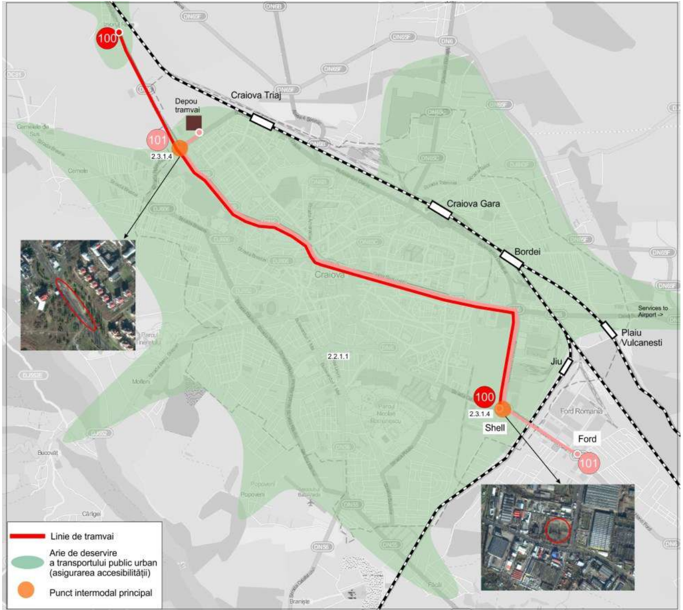
Figura 121: Măsurile propuse pentru operarea transportului public în municipiul Craiova, Scenariul 1 (linii principale)
