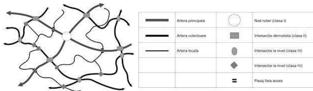
Figura 125: Planificarea tramei stradale după funcția străzilor (Sursă: Normativ pentru amenajare intersecții la nivel pe drumurile publice, indicativ AND 600)
