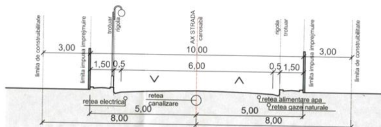
PROFIL STRADAL TRANSVERSAL
