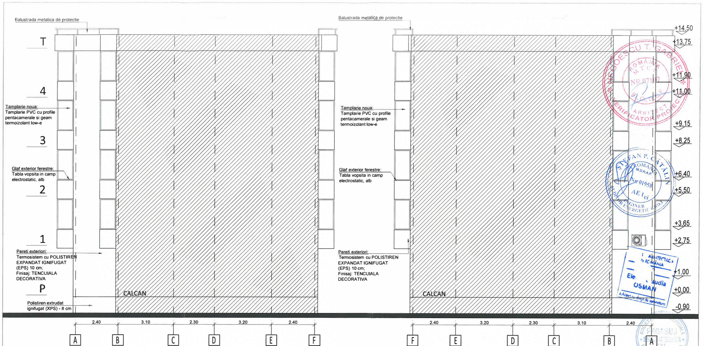
FATADA SUD-VEST
