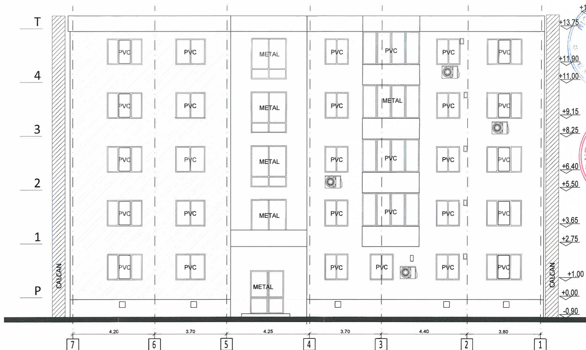
FATADA SUD-EST
