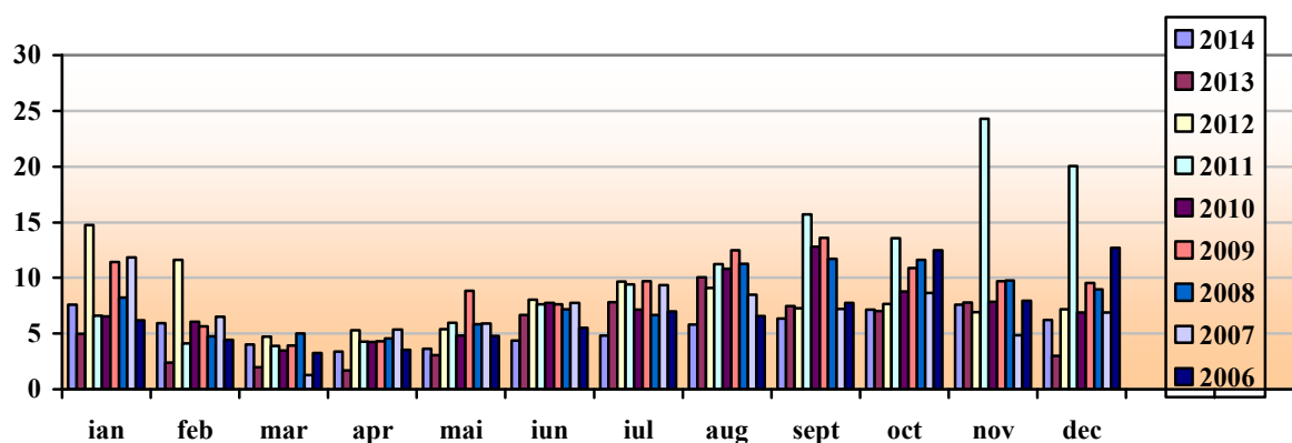
e. Evoluția radioactivității descendenților radonului, în ultimii 9 ani, aspirația între orele 20-01
